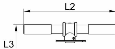
Poignée DN65 - 100 (2"1/2 - 4")
